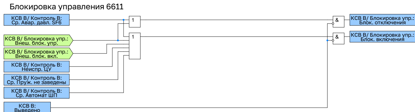
Рисунок 2.51 – Функциональная схема логики блокировки управления выключателя
