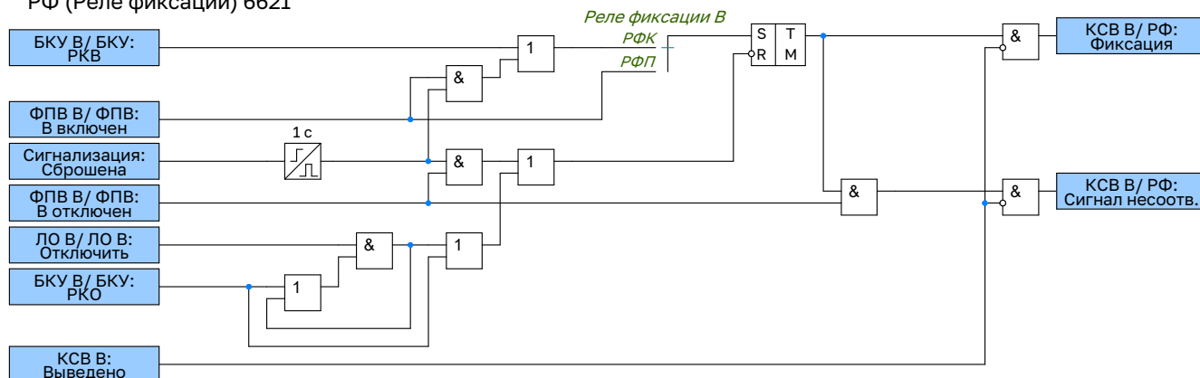
Рисунок 2.52 – Функциональная схема логики реле фиксации выключателя
