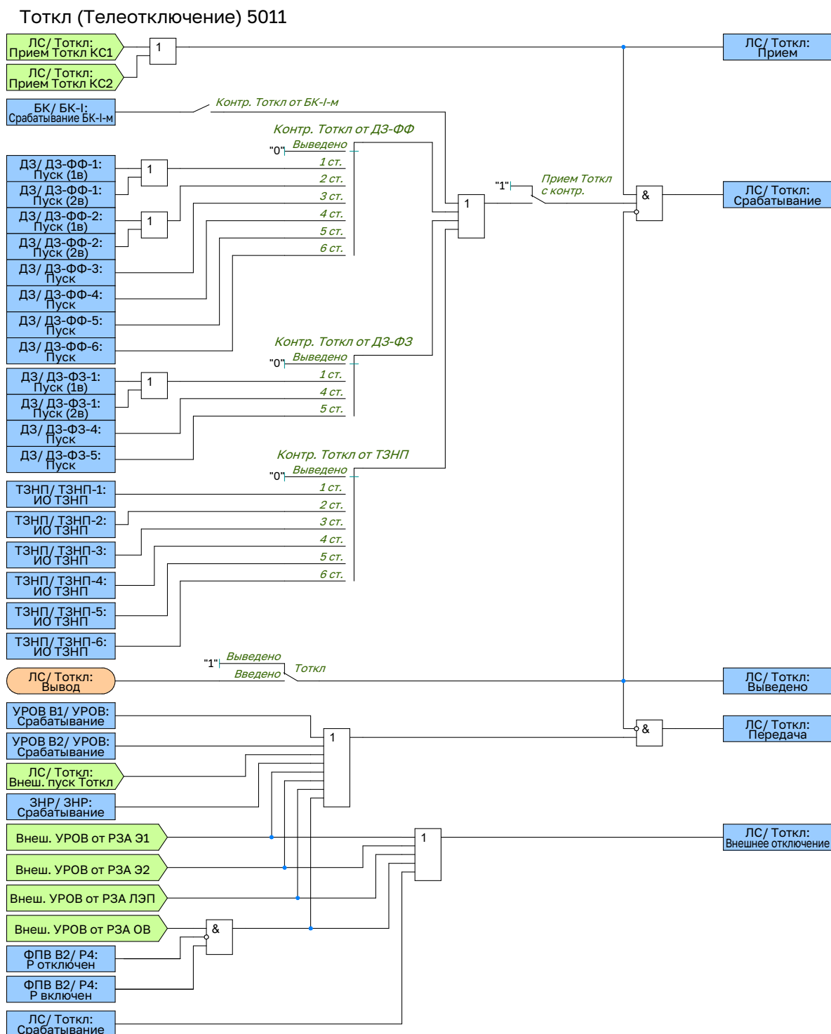
Рисунок 2.37 – Функциональная схема логики телеотключения
