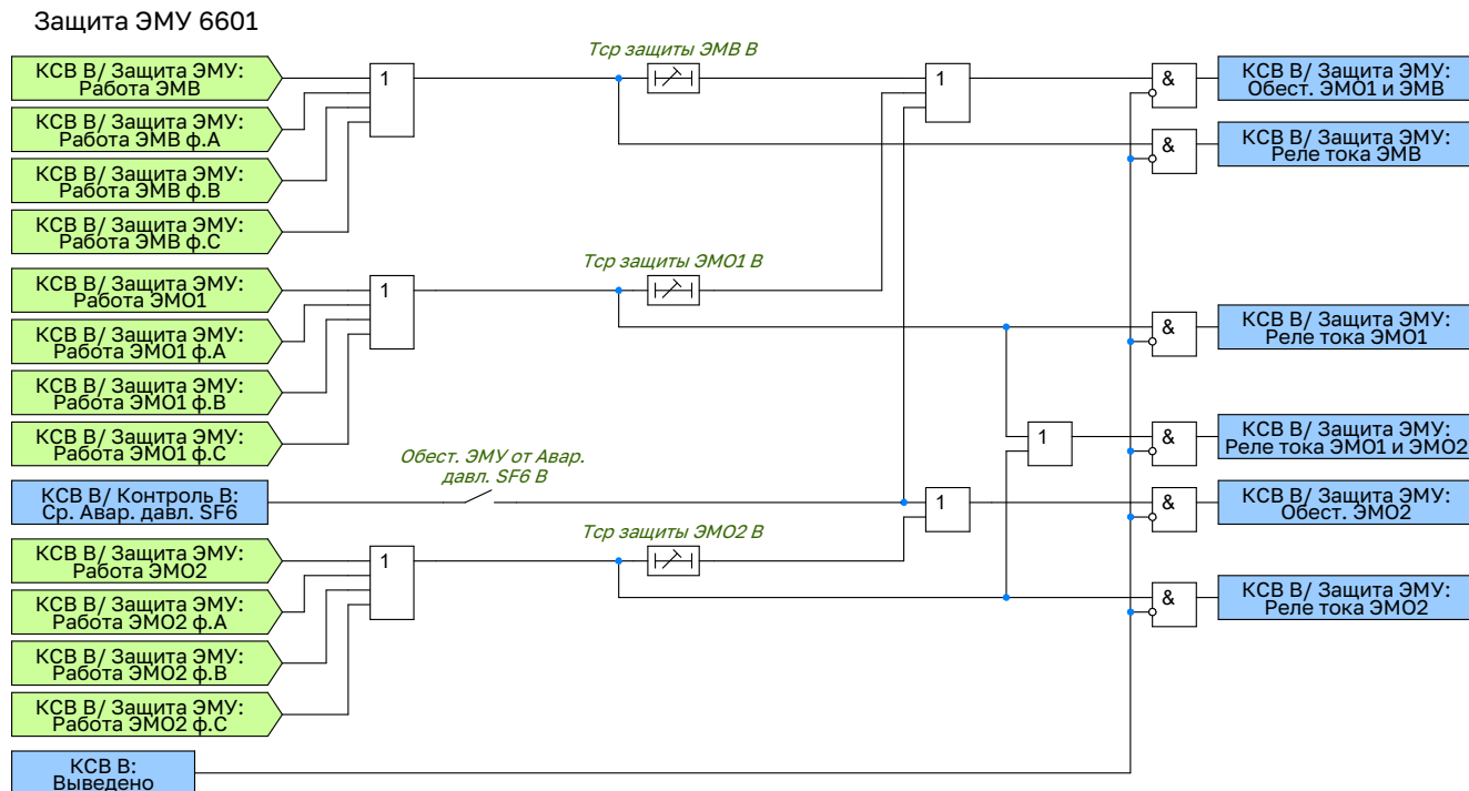
Рисунок 2.50 – Функциональная схема логики защиты ЭМУ выключателя
