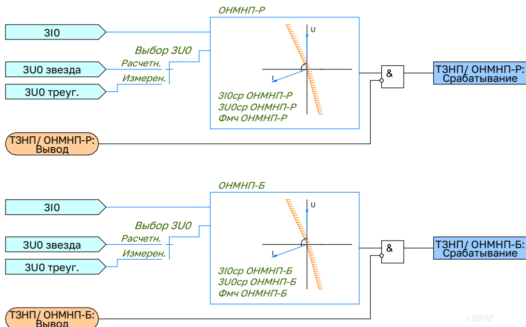
Рисунок 2.23 – Функциональная схема логики OНМНП
